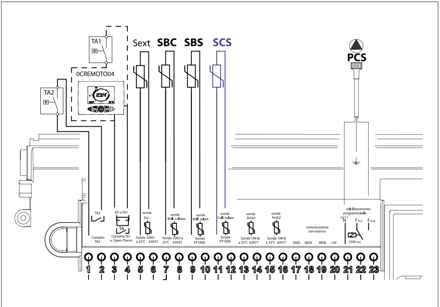
Рис. 26 Подробная электрическая схема Модель KRBS
