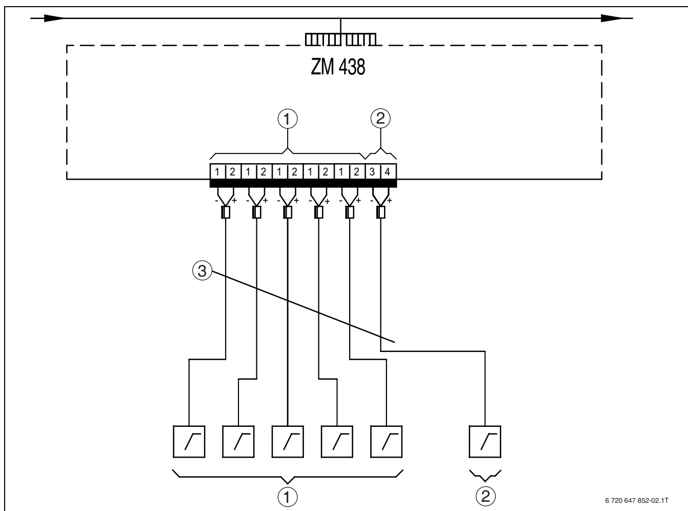
23 pav. Jungimo schema ZM 438
