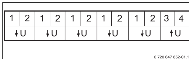
Rys. 28 Wejścia i wyjścia ZM 438
