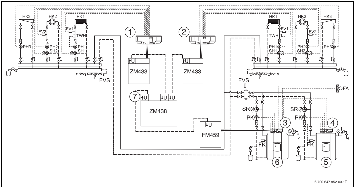
Fig. 6 Esempio d'impianto
