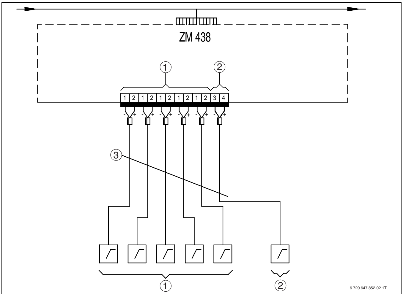
Bild 2 Schaltbild ZM 438
