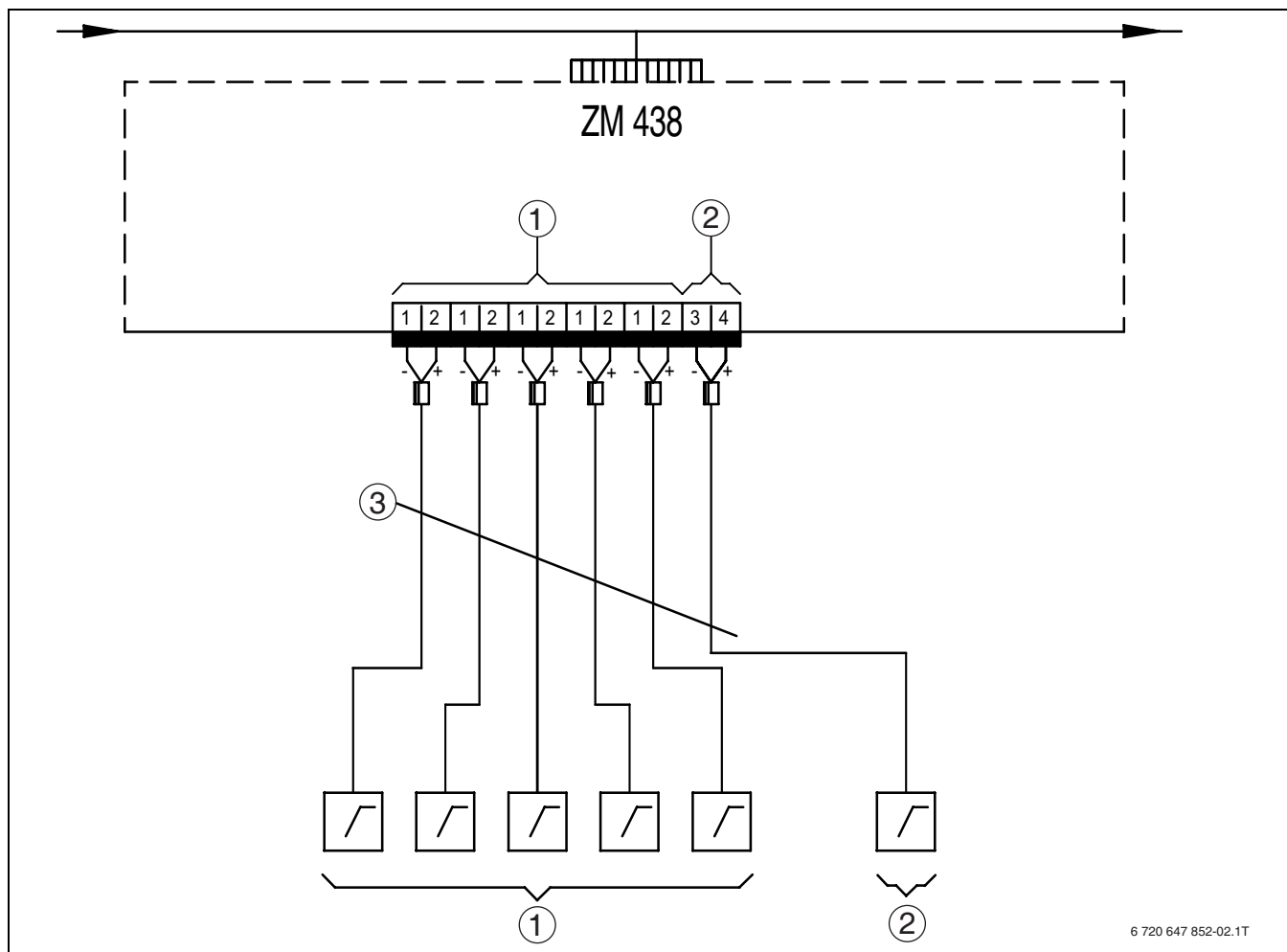
Σχ. 11 Διάγραμμα συνδεολογίας ZM 438
