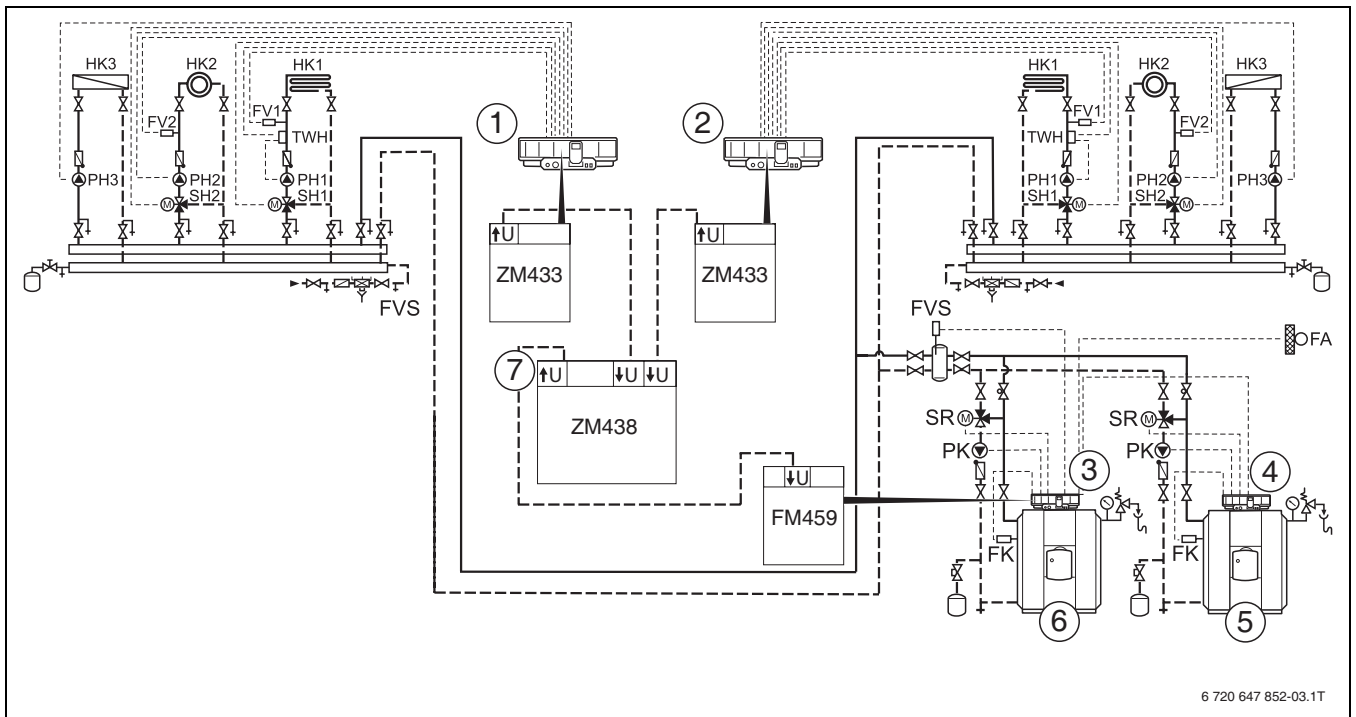
Σχ. 12 Παράδειγμα εγκατάστασης
