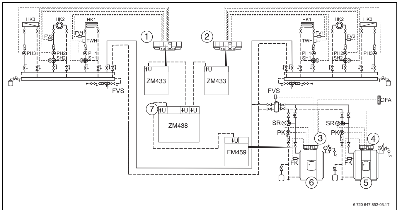
Фиг. 9 Пример за инсталация
