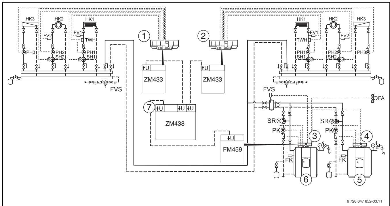
Рис. 33 Пример установки
