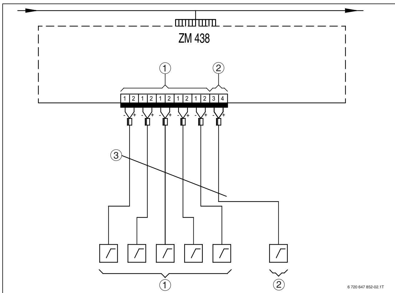
Rys. 29 Schemat ZM 438
