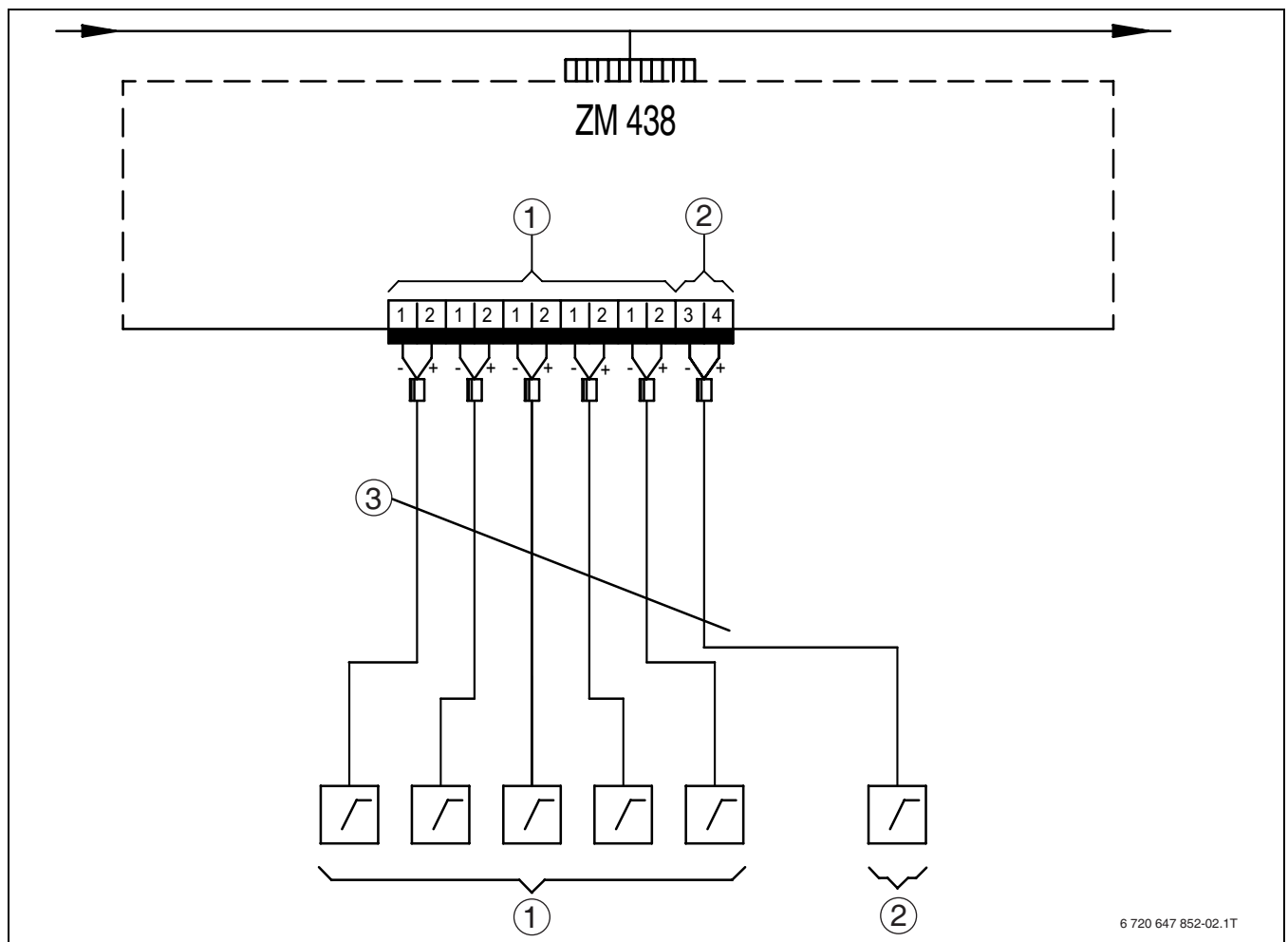
Фиг. 8 Електрическа схема ZM 438
