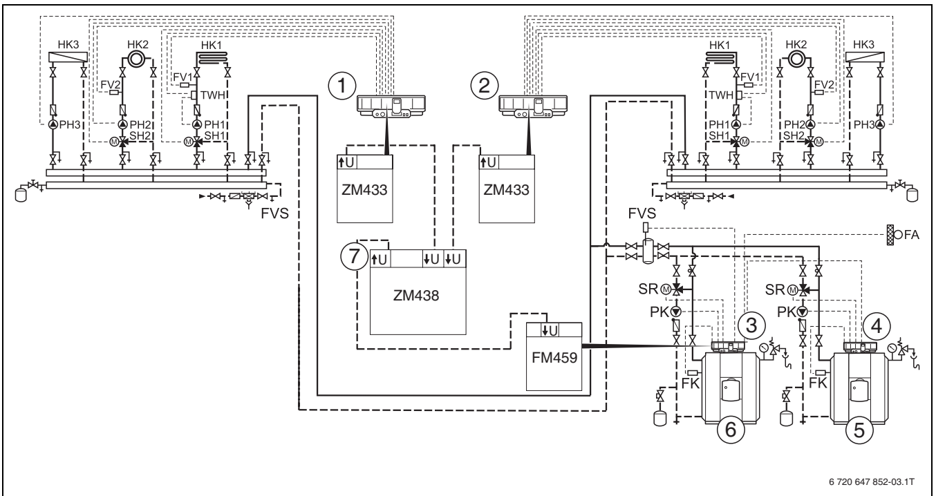
24 pav. Įrenginio pavyzdys
