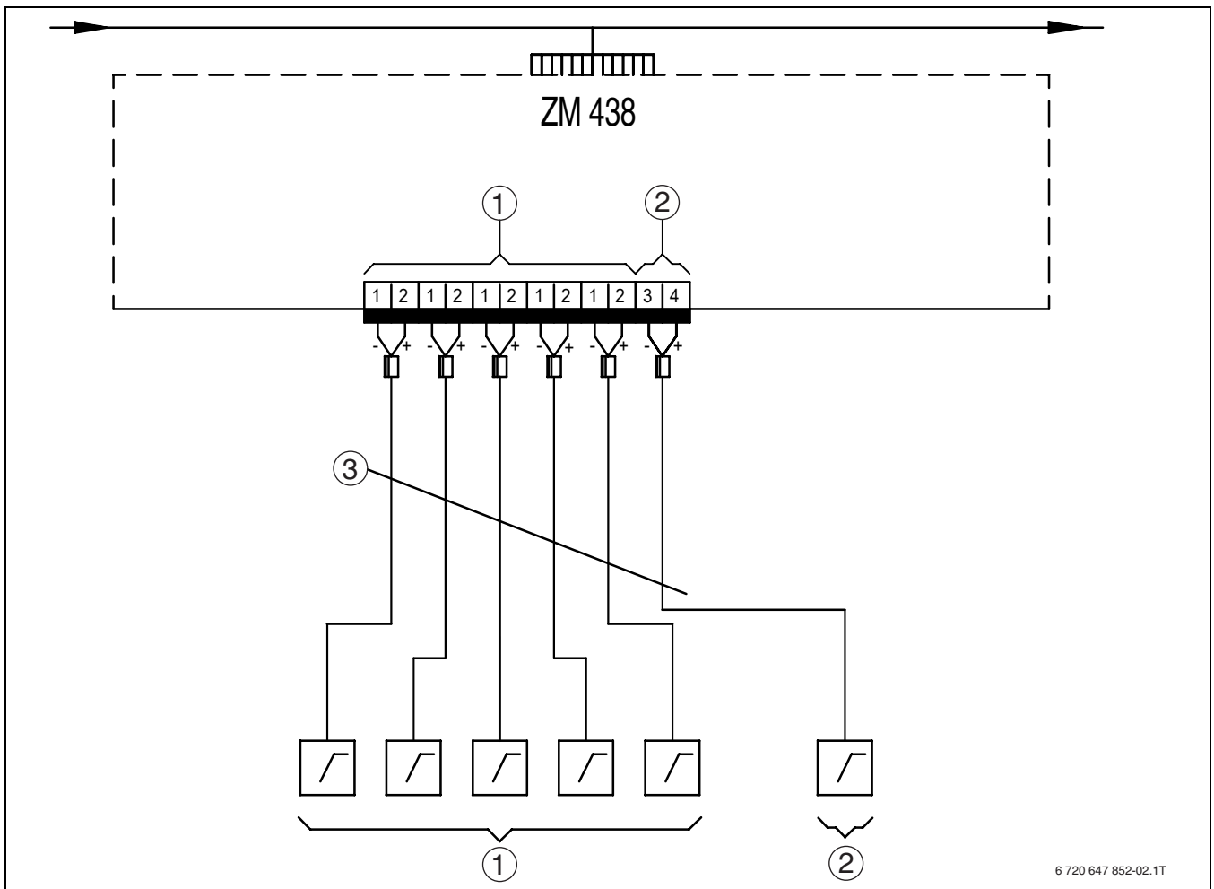
26. att. ZM 438 pieslēgumu shēma
