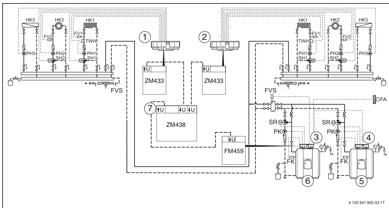
Мал. 39 Приклад інсталяції
