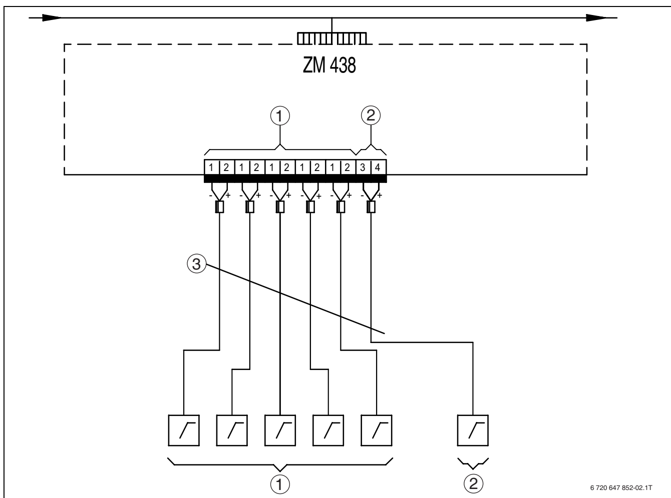
Joon. 14 ZM 438 ühendusskeem
