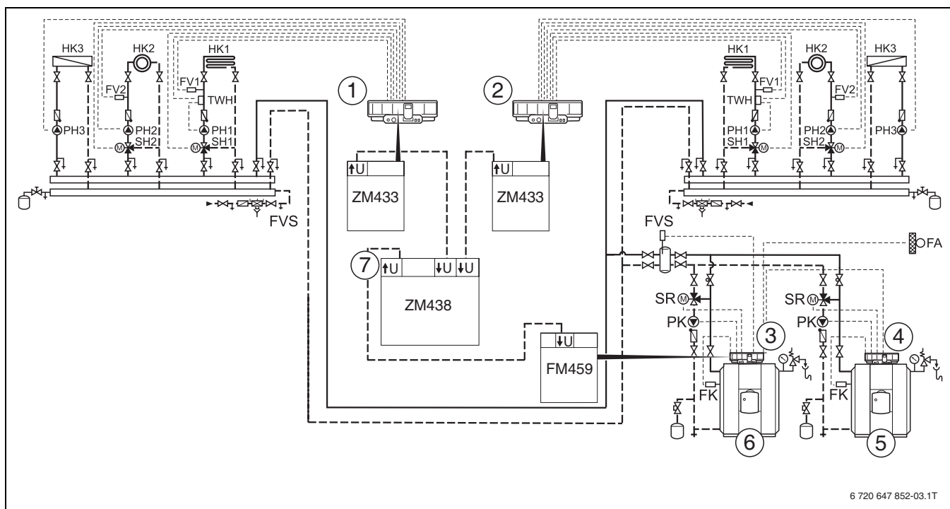
Sl. 18 Primjer instalacije
