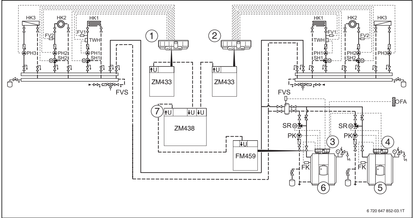
Res. 36 Tesisat örneği
