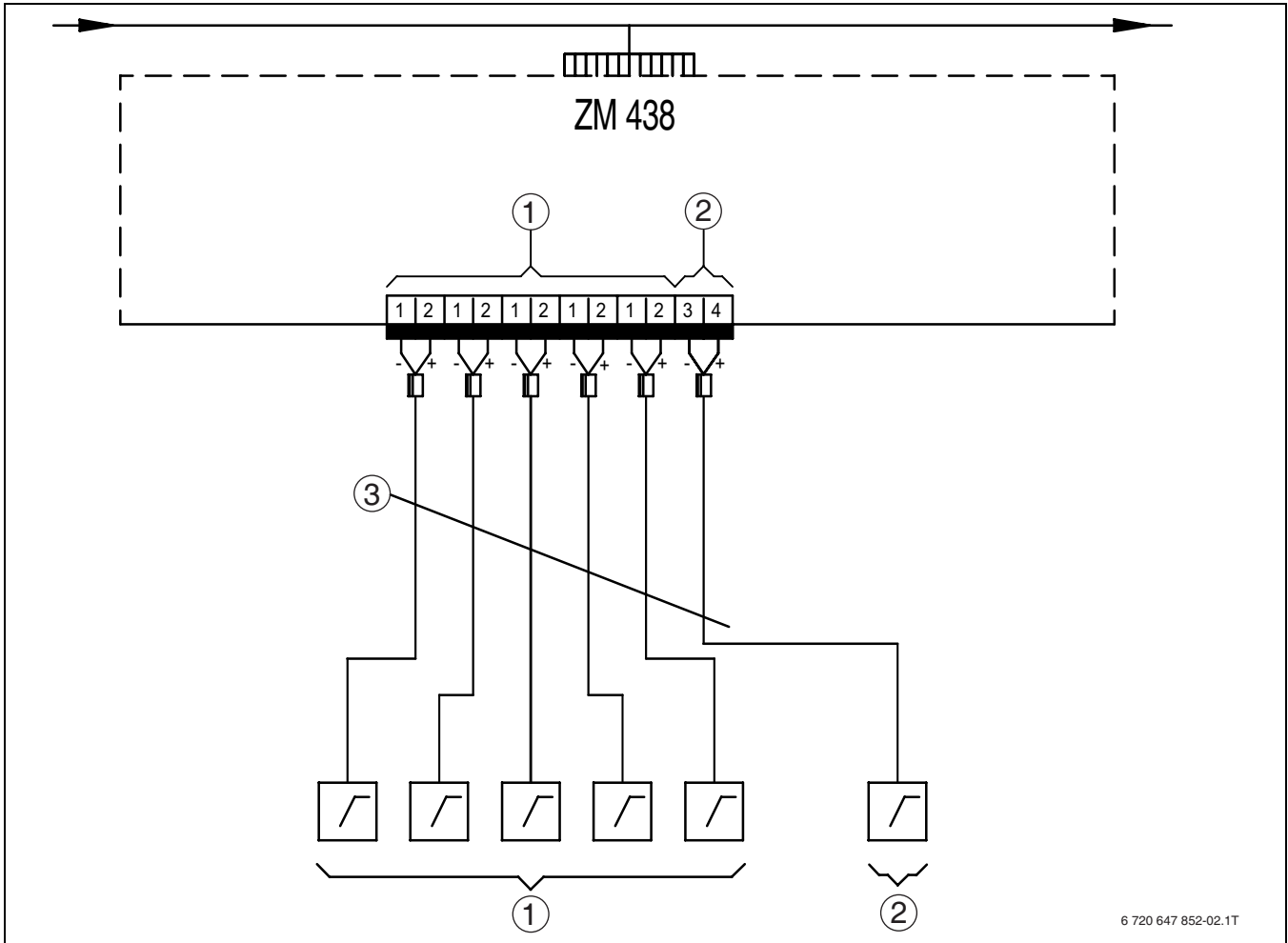
Res. 35 ZM 438'in devre şeması
