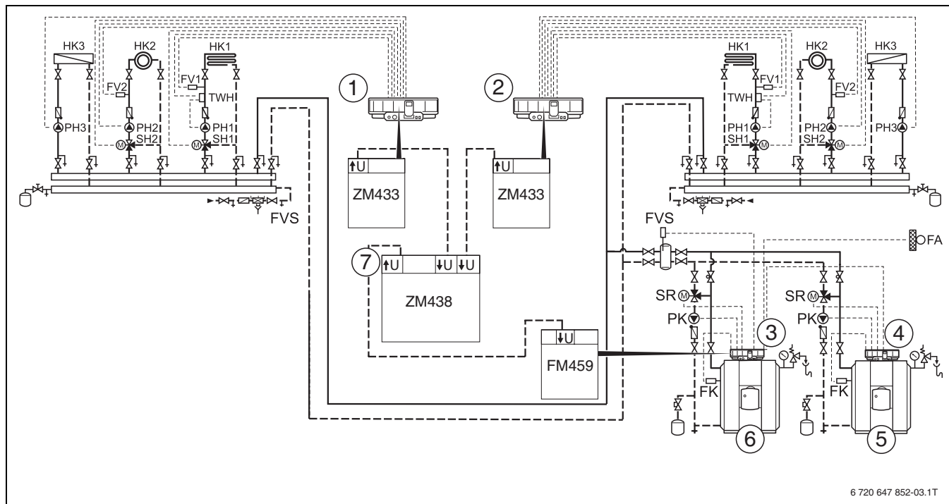
21. ábra Rendszerpélda
