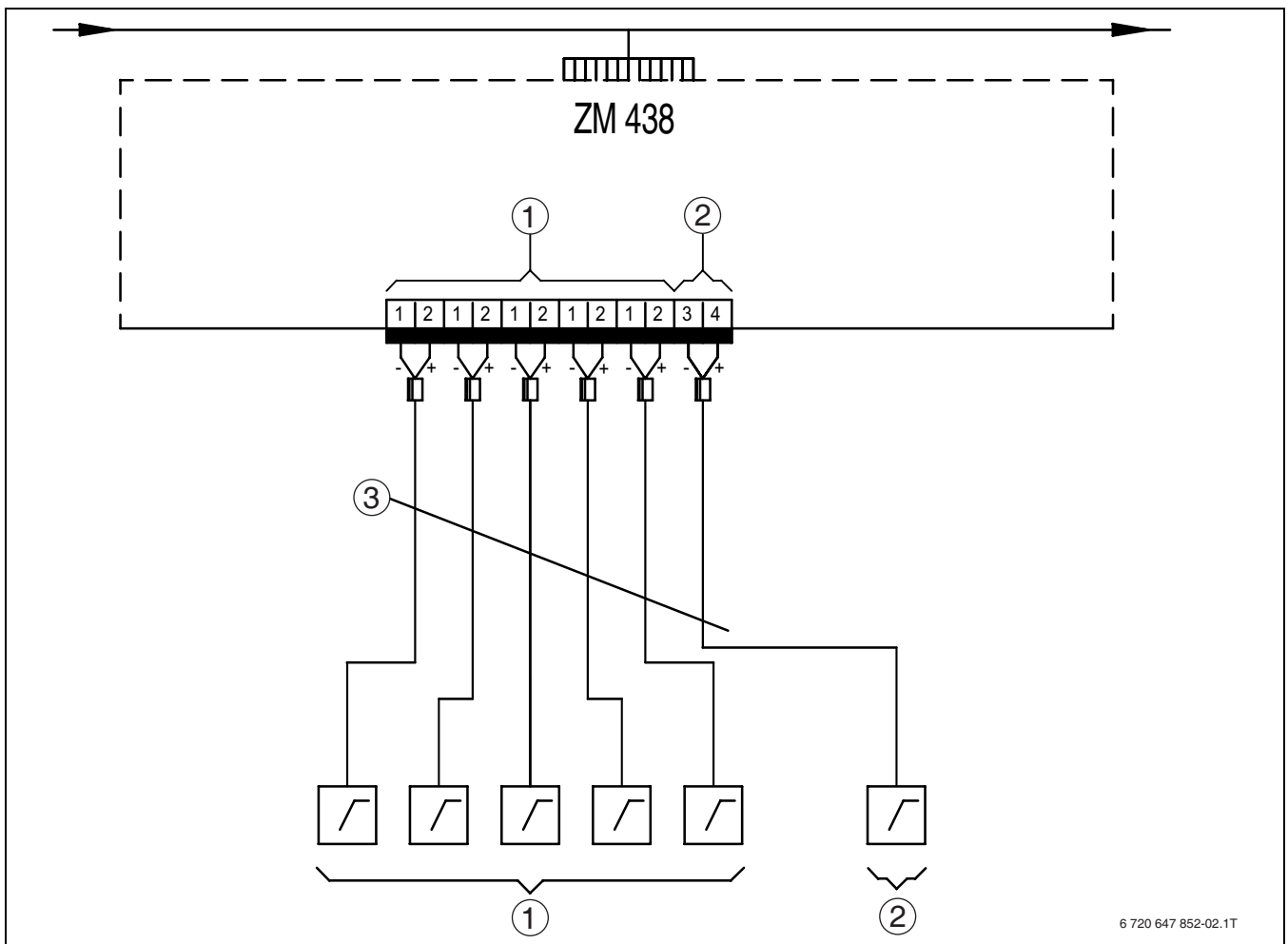
Мал. 38 Схема електричних з'єднань ZM 438
