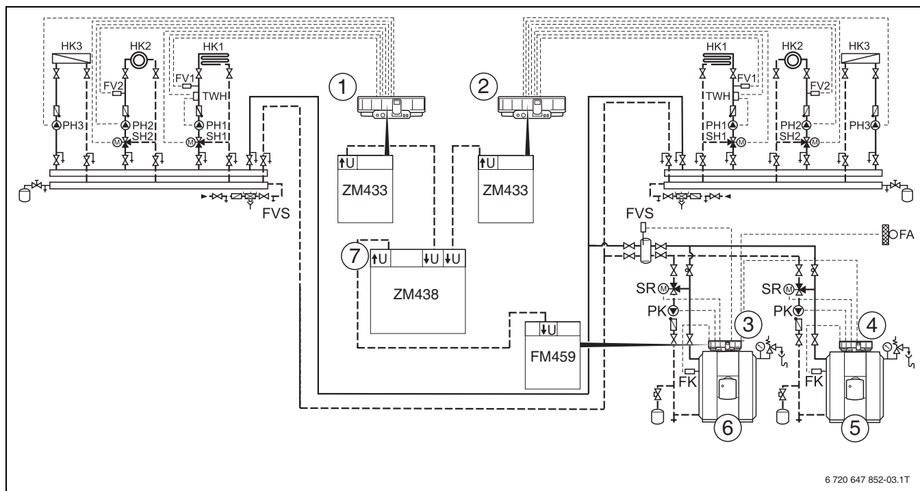
27. att. Sistēmas piemērs
