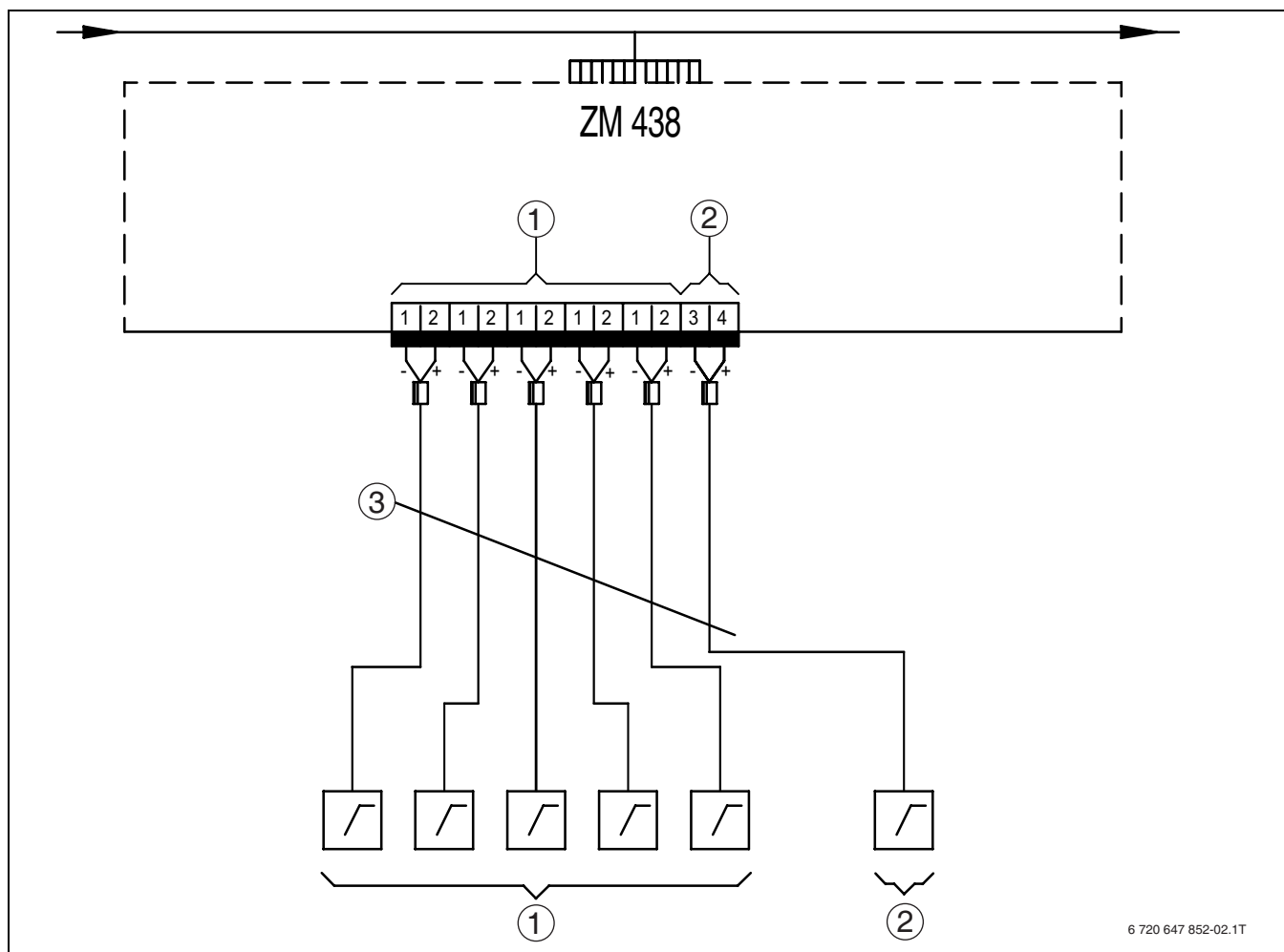
Sl. 17 Spojni dijagram ZM 438
