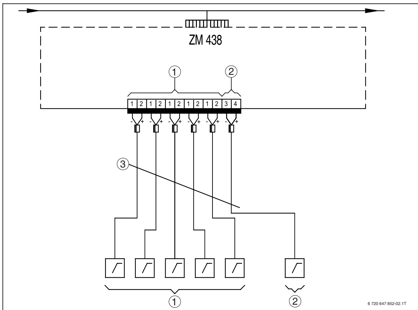
Fig. 5 Schema elettrico ZM 438
