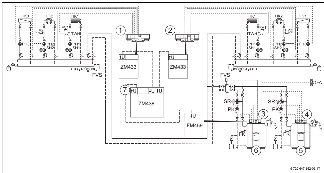
Joon. 15 Süsteemi näide
