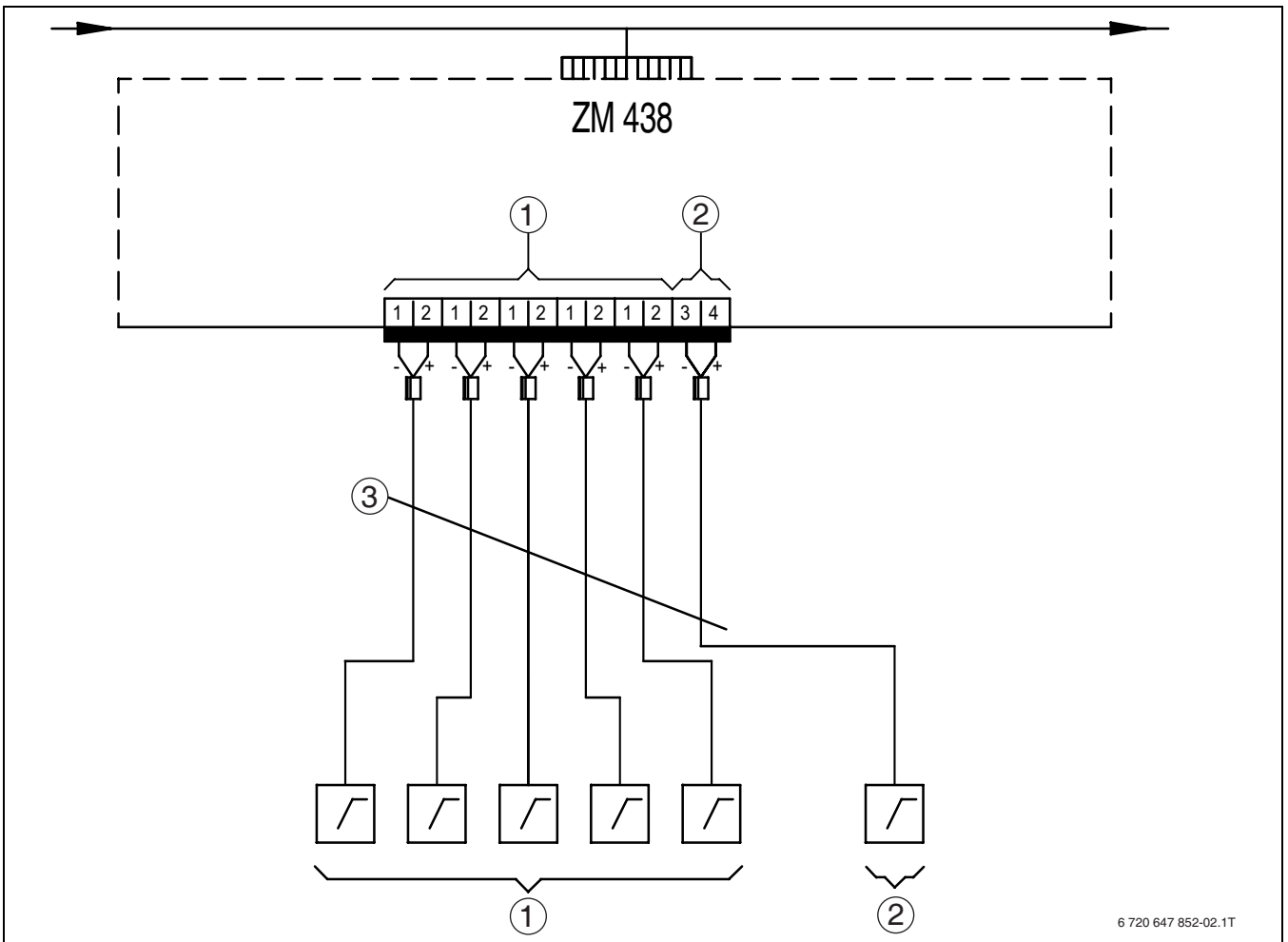
Рис. 32 Электрическая схема ZM 438
