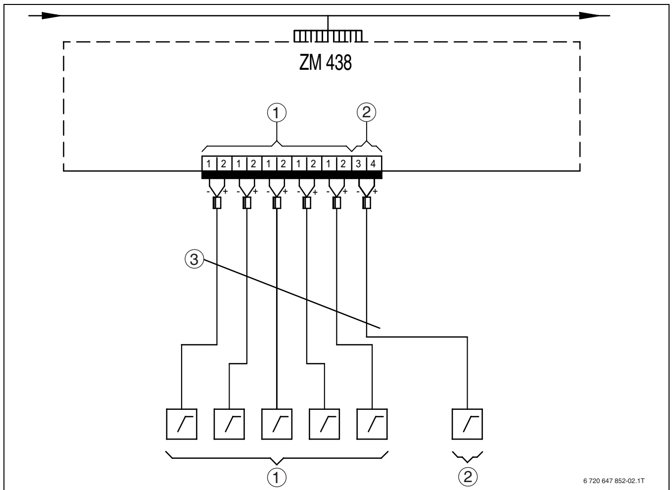
20. ábra A ZM 438 kapcsolási rajza
