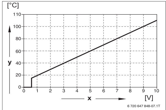
Рис.13 Вход 0 – 10 В
