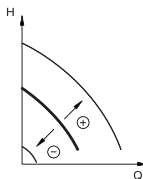
15-сур. Тұрақты сипаттамалы басқару режиміндегі сорғы
