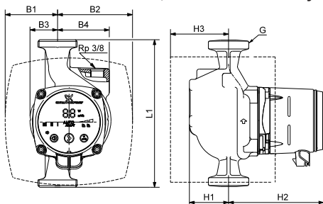
30-сур. ALPHA3 25-40 A, 25-60 A
