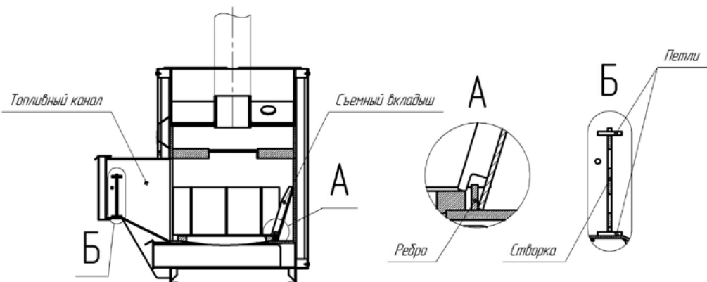
Рис. 56. Установка заднего вкладыша под уголь и створки в топку печи
