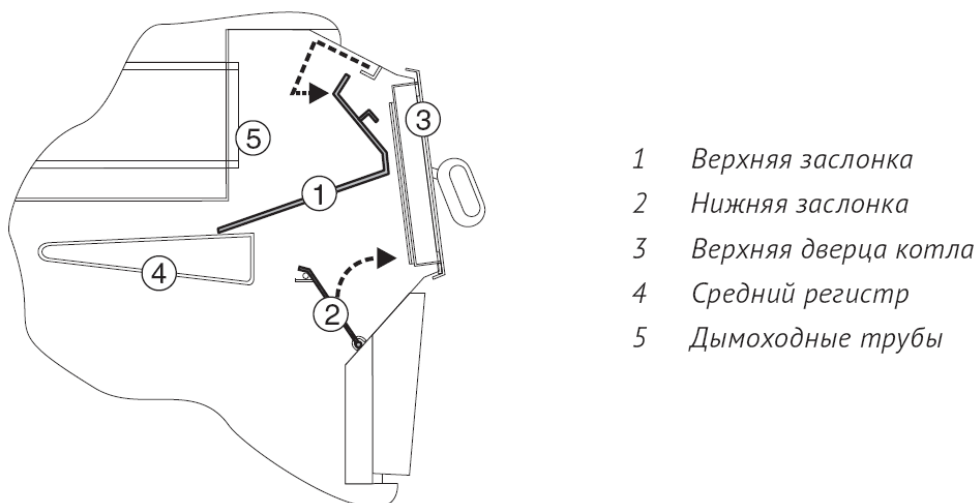
Рисунок 11. Снятие подвижных заслонок из камеры сгорания
