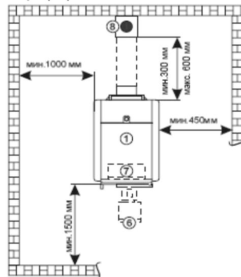
Рисунок 2. Минимальные расстояния от котла до стен котельной
